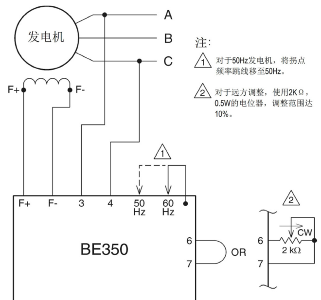
图1 - BE350典型接线
